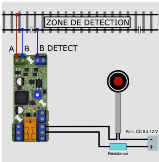
Figure 2. Schéma de câblage d'un feu clignotant avec alimentation par courant continu (valeur de la résistance adaptée à la tension du courant).
