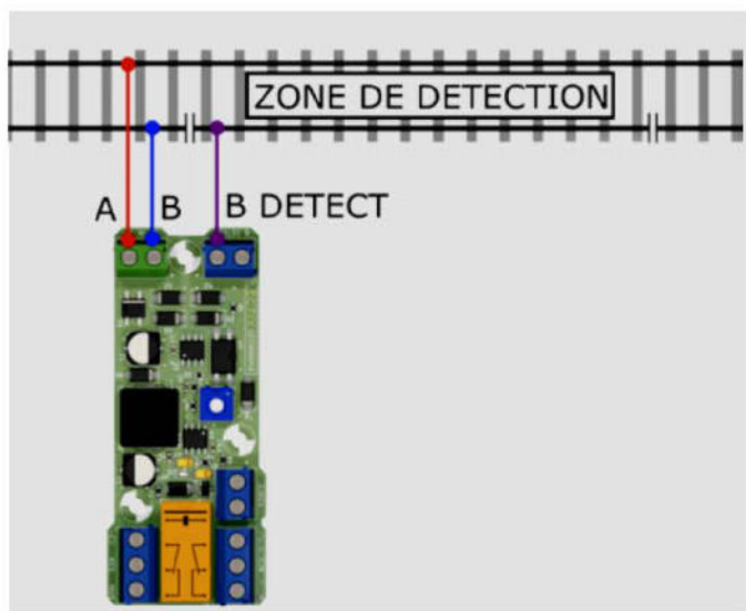
Figure 1. Schéma de câblage de la détection par consommation de courant (document Lectix). Dans le cas d'un passage à niveau sur voie unique, la zone de détection est étendue de part et d'autre du PN, légèrement plus longue que le plus long des convois empruntant la ligne.
