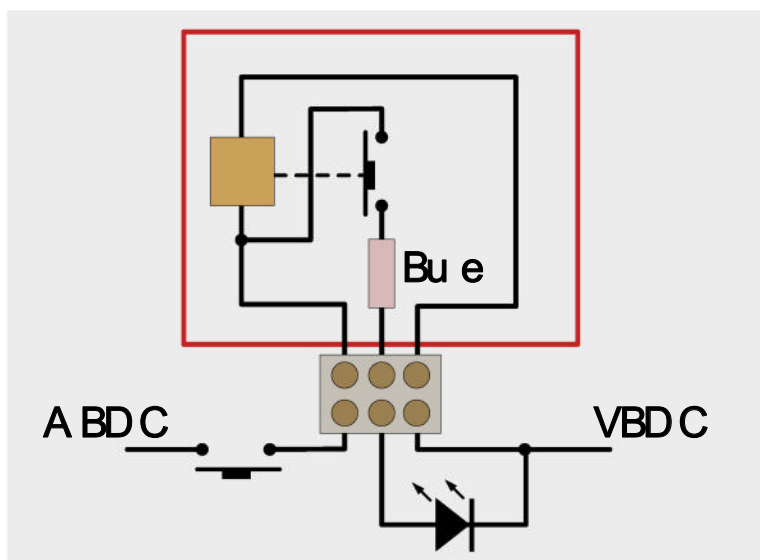
Figure 1. Schéma de câblage
