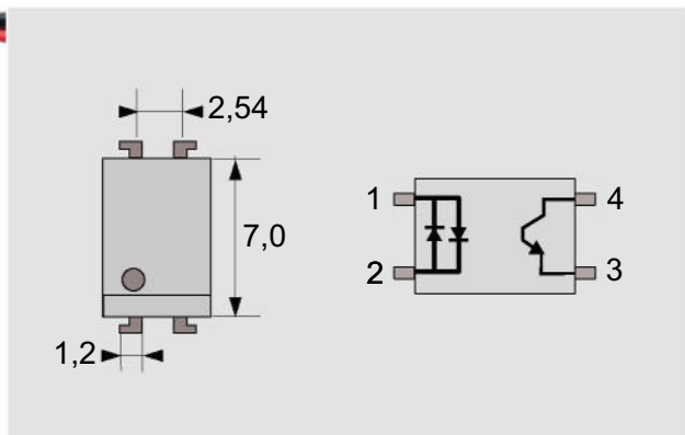
Figure 2 Schéma de brochage de l'opto-coupleur ISP814X Farnell.
