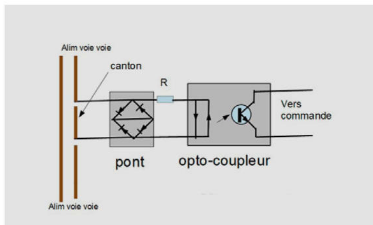
Figure 1 Schéma de branchement du détecteur.
