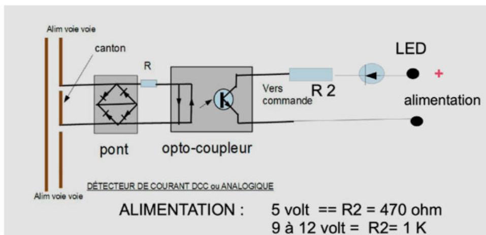
Figure 1 Schéma de branchement du détecteur.
