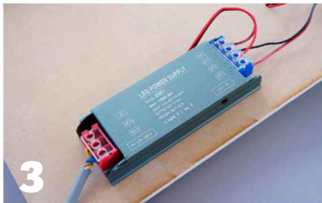
Le transfo nécessaire aux rubans à LED, autres que ceux alimentés directement en 220 V, est fixé dans l'angle arrière gauche. N'hésitez pas à prendre un transfo d'assez bonne qualité, les LED peuvent griller plus rapidement avec un transfo de bas de gamme.
