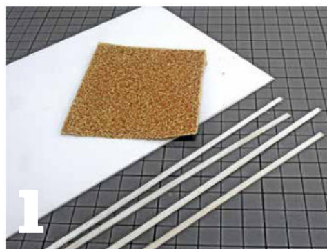
Figure 1 Schéma d'assemblage. Les poteaux, les planches et les traverses sont découpés dans de la carte plastique en plaque. L'utilisation de profilés déjà aux cotes est possible mais serait plus onéreuse.
