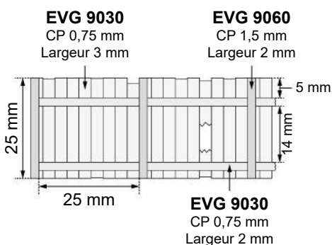
Figure 1 Schéma d'assemblage. Les poteaux, les planches et les traverses sont découpés dans de la carte plastique en plaque. L'utilisation de profilés déjà aux cotes est possible mais serait plus onéreuse.
