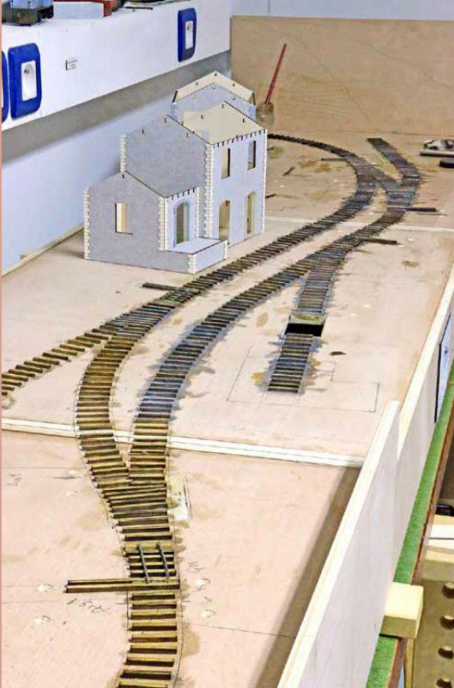
Le travelage en bois est rapidement posé grâce à l'emploi de gabarits découpés au laser.
