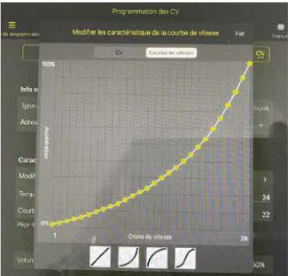
1. Lecture et affichage de la courbe d'usine.
