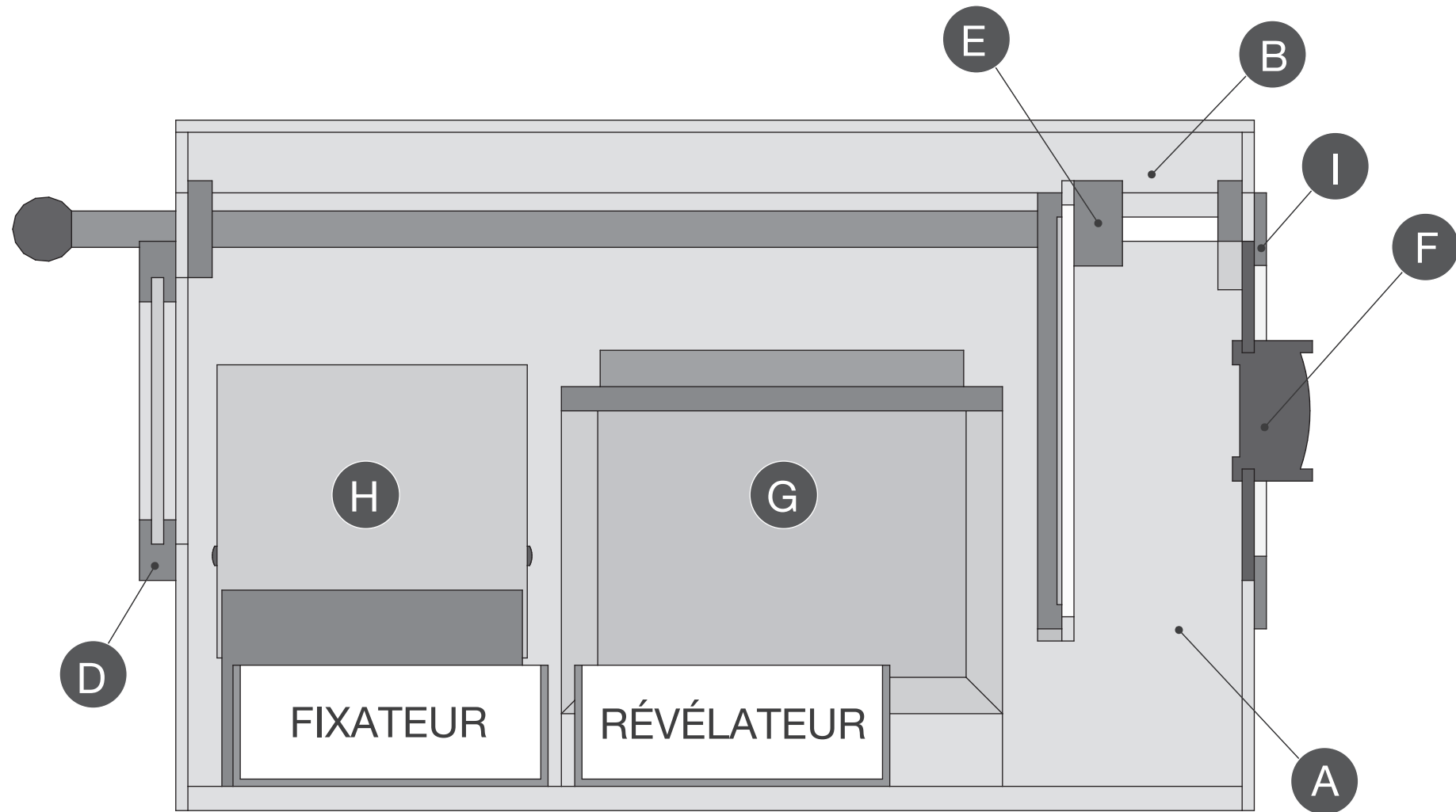
Coupe longitudinale
