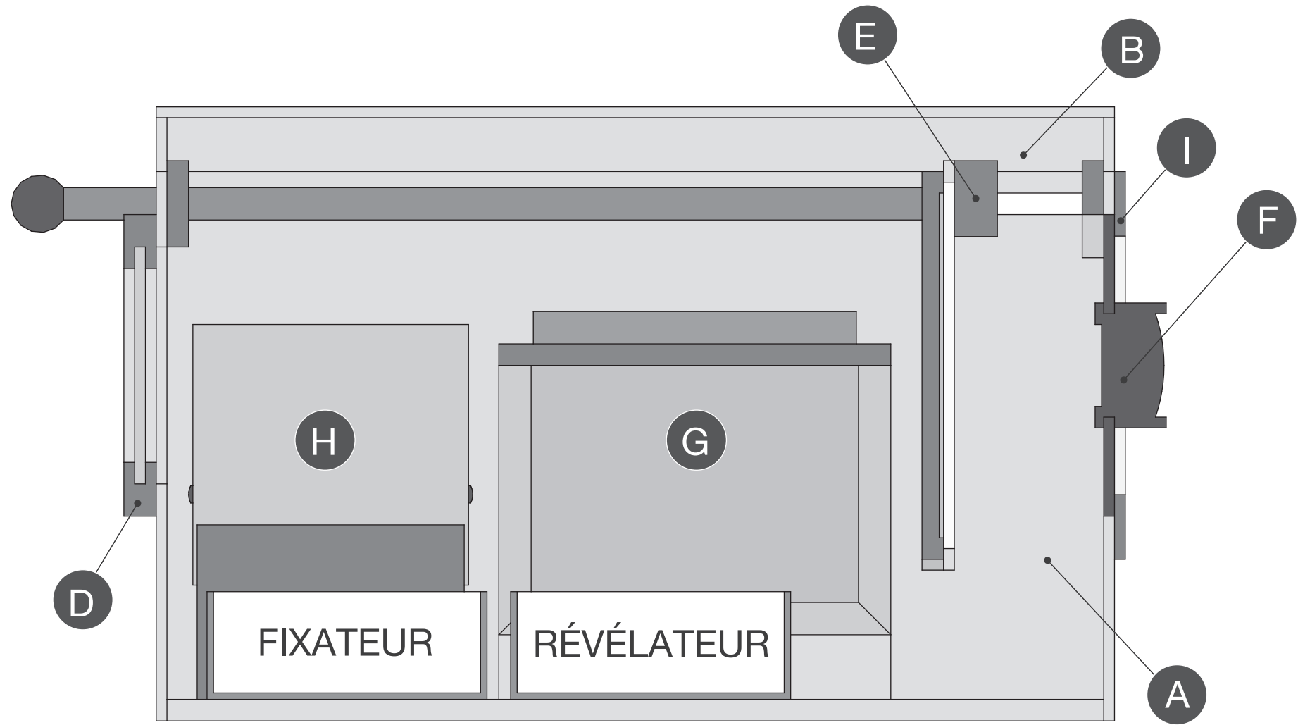
Coupe longitudinale
