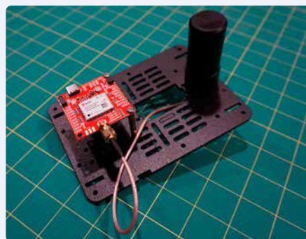
Figure 3. La carte GPS montée sur un châssis séparé, installée au-dessus de la Jetson Nano et de la montage de la caméra.
