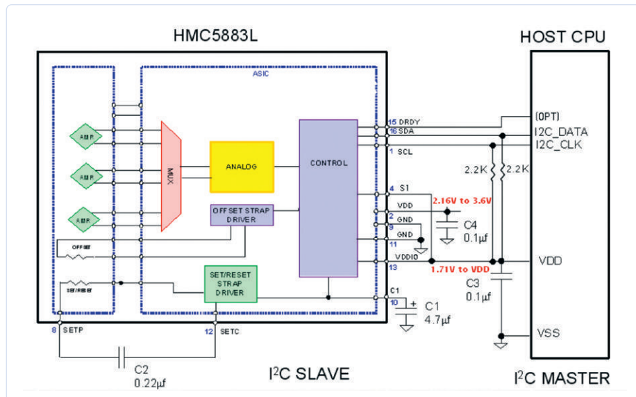
Figure 1 : Circuit interne du capteur boussole HMC5883L (source : fiche technique Honeywell).
