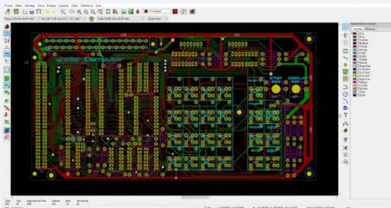
Figure 3. Reconstruction du circuit sous KiCAD.
