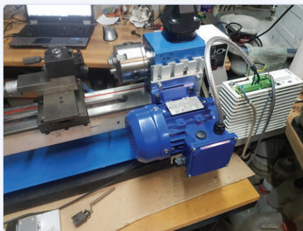
Figure 7. Montage du moteur de 0,37 kW et du variateur.
