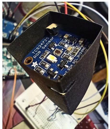
Figure 4. Capteur RVB TCS34725 avec son écran de protection noir.
