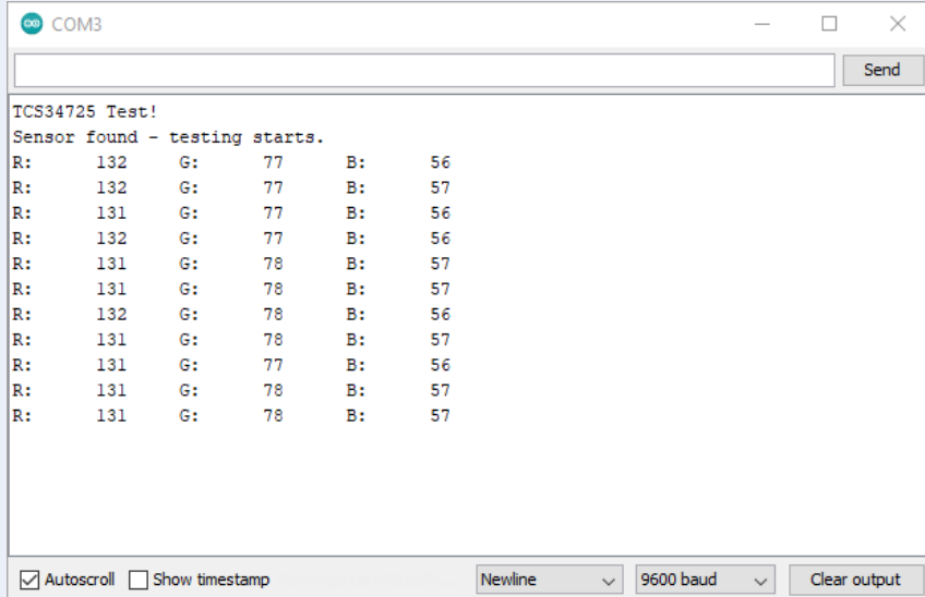
Figure 3. Sorties de valeurs RVB fournies par le croquis tcsrgbsensor.ino Arduino.
