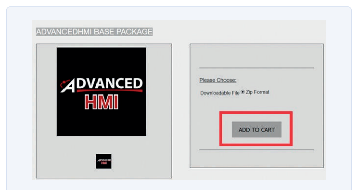
Figure 2. Téléchargement d'AdvancedHMI.
