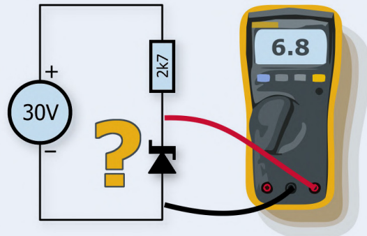
Figure 1. Une façon de tester rapidement les diodes Zener.
