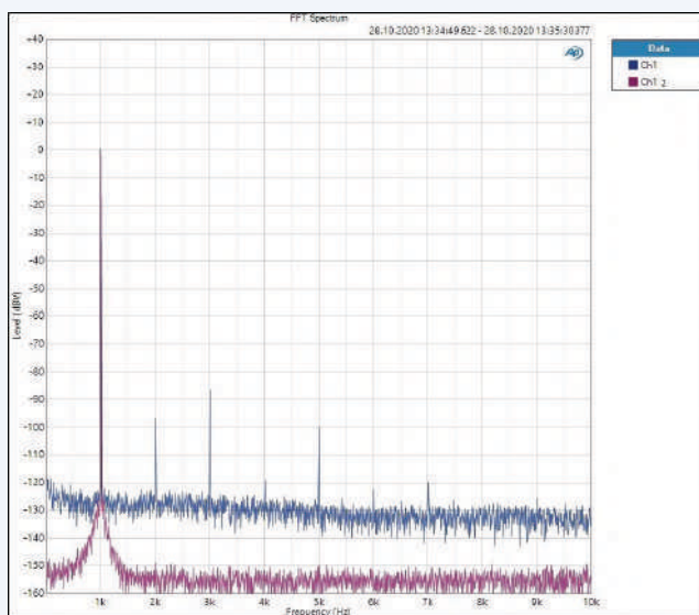
Figure 2. Comparez avec la figure 1. Spectre d'une onde sinusoïdale, 1 kHz, 1 V_{\text{eff}} avec le Steinberg UR22.
