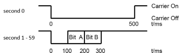
Figure 10. L'impulsion des secondes MSF montrant le codage Bit A et Bit B.
