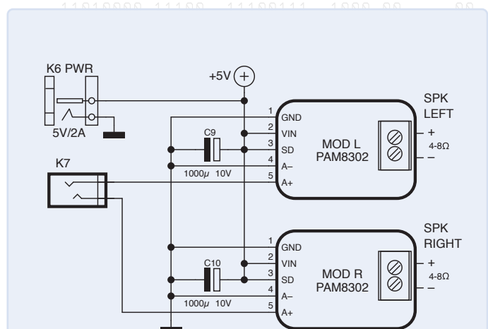
Figure 3. Schéma de la carte d'amplification optionnelle.
