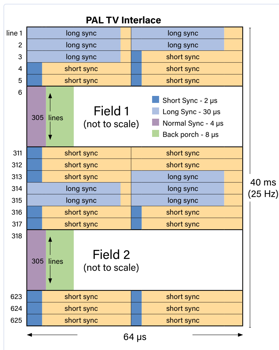
Figure 7. Composition d'une image PAL complète. (Source : martin.hinner.info)
