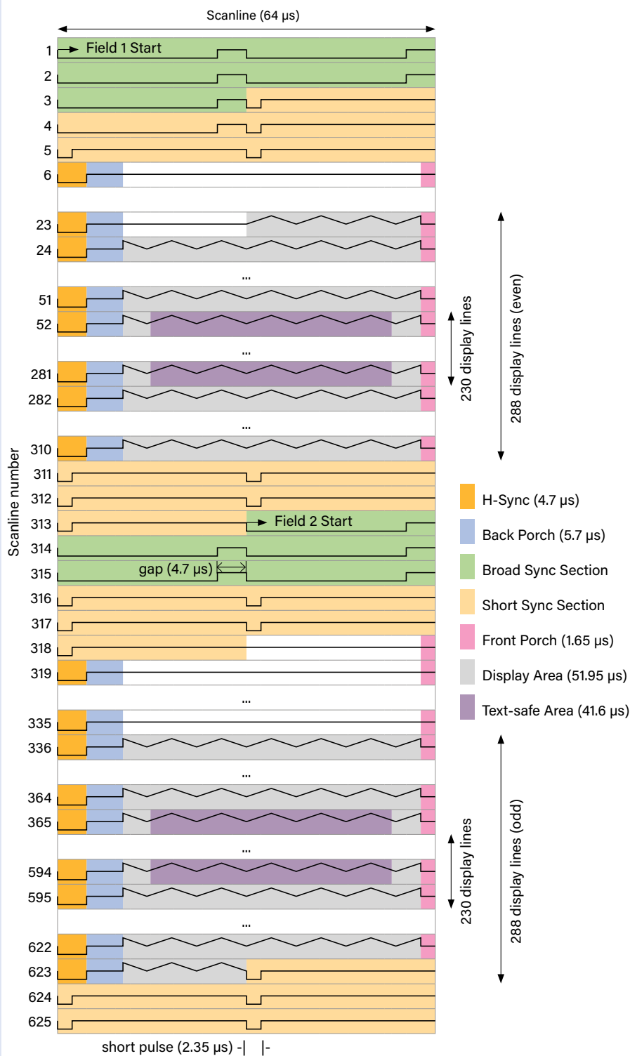
Figure 19. Signal de sortie d'image avec une demi-ligne de trame. (Source : batsocks.co.uk/https://tinyurl.com/4fyghmk)
