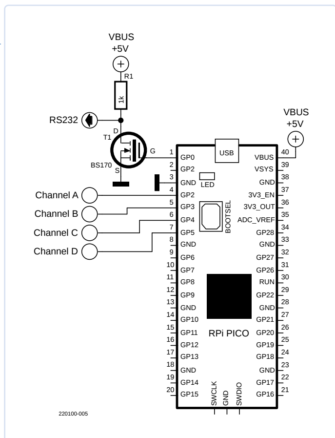
Figure 4. Connexion d'un oscilloscope à quatre canaux au RPi Pico pour visualiser les formes d'onde de sortie du premier exemple.
