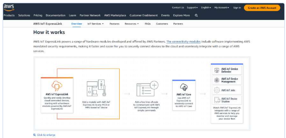
Figure 3. ExpressLink est un module de connectivité qui fournit une interface de commande AT simple au microcontrôleur hôte.
