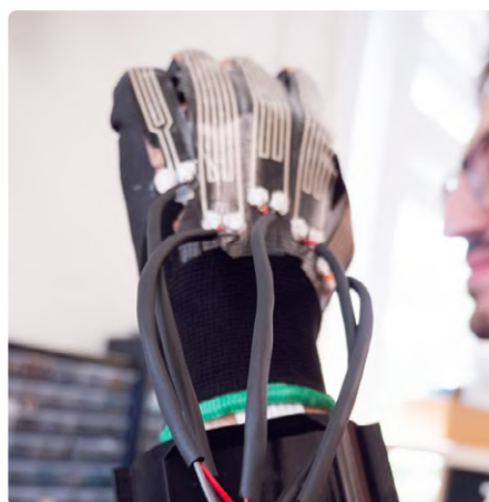
Figure 6. En exploitant les variations de résistance de l'encre conductrice sur un substrat extensible, les jauges de contrainte situées dans les doigts de ce gant pourraient contrôler une main robotisée.
