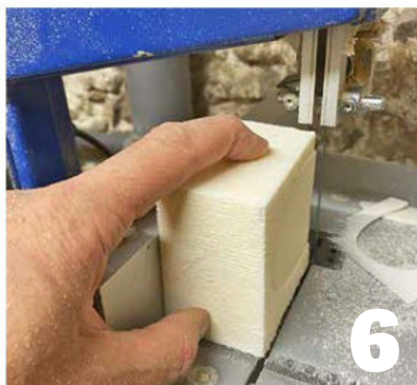
En inclinant le plateau de la scie à ruban, on découpe chaque section selon l'angle choisi.
