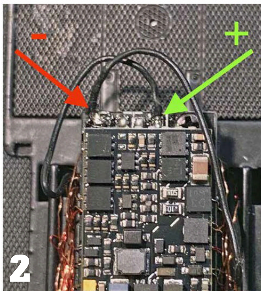
Branchement du détecteur sur le décodeur.
