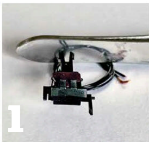
La tête d'attelage Krois et ses deux fils de commande.
