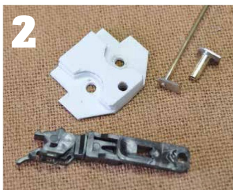
2 L'embase (vue de dessous). L'assise des vis de fixation sur le bogie est telle que les têtes ne dépasseront pas du plan sur lequel sera positionné le timon. Les plaquettes, l'une avec un tronçon de tube, l'autre munie d'un rond.
