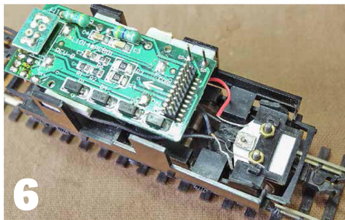
6 Le timon installé; les composants électriques ne sont pas encore reposés.
