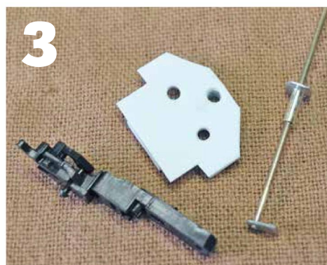
3 À côté de la face de l'embase qui prendra appui sur le bogie : le montage à blanc des plaquettes.
