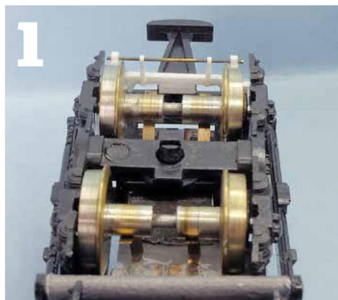
Vue de dessous du châssis et du bogie arrière, caisse démontée. Il va falloir passer au milieu de tout cela!
