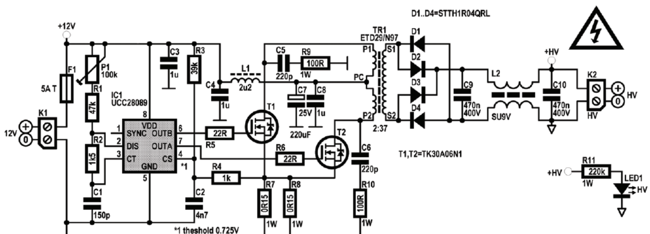
Figure 1. Schéma de principe du convertisseur CC/CC.
