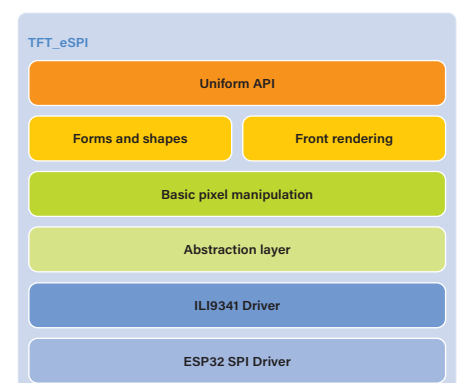
Figure 5. Fonctions de dessins empilées pour l'écran LCD.
