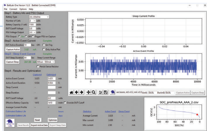
Figure 6. Trace montrant le courant circulant dans une résistance de 1 k \Omega sous 3 V avec un certain niveau de bruit apparent.
