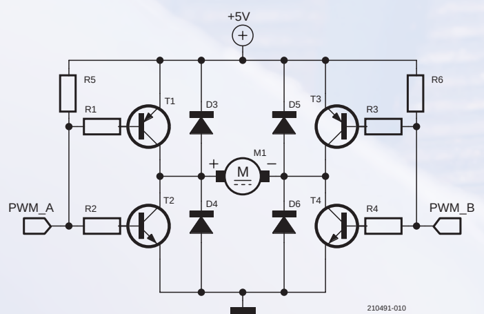
Figure 6. Commande par signaux MLI provenant \mu C .
