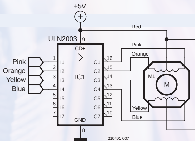
Figure 18. Schéma du circuit avec ULN2003 et moteur pas à pas.
