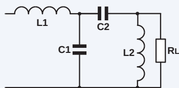
Figure 1. Filtre passe-bande.
